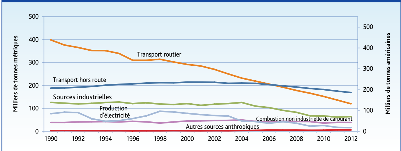
Figure 18. Tendances des émissions canadiennes de \text{NO}_x dans la ZGEP, 1990 à 2012
